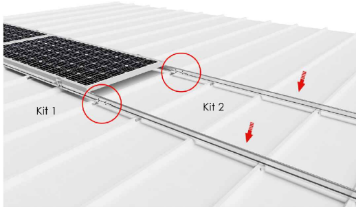
Kit 1 - Fijar las uniones del perfil guía mediante tornillos de unión Kit 2 - Colocar los perfiles del nuevo kit en las uniones y fijarlas con los tornillos de unión
